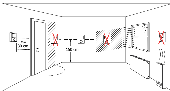
Рисунок 31. Положение термостата
