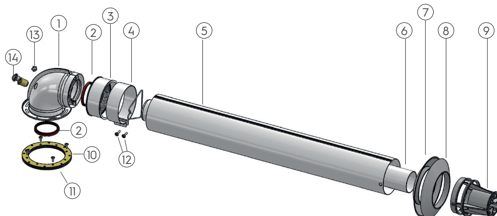
Рисунок 11. Дымоход котла
