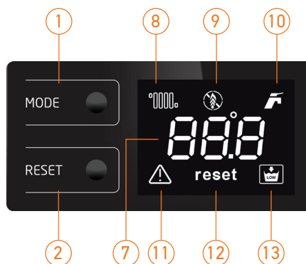
Рисунок 27. Экран автоматической панели управления LAWA SMART
