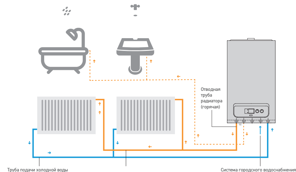
Рисунок 24. Общая схема монтажа
