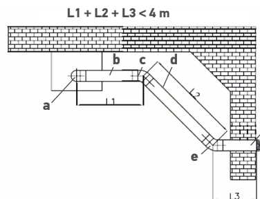
Рисунок 17 III. Монтаж дымохода с двумя отводами 45° и одним отводом 90°.
