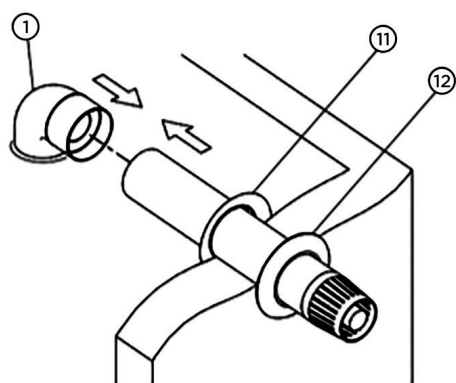
Рисунок 12 Выход дымохода в стене
