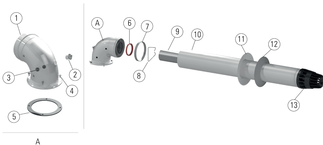
Рисунок 11. Дымоход котла
