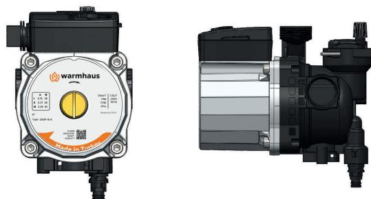
Рисунок 23. Насос с автоматическим краном выпуска воздуха и 3 уровнями скорости
