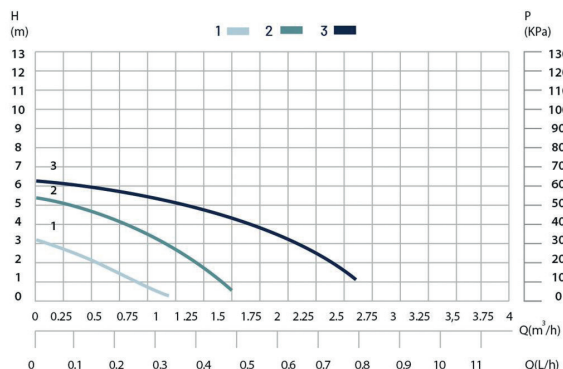
Рисунок 22. Кривая потока / давления насоса
