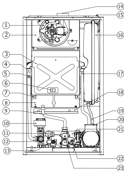
Рисунок 25. Компоненты котла
